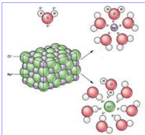
Figura 2.12. Tretësi e klorurit të natriumit dhe hidratimi i joneve të tij.
