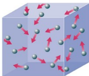
Fig. 3.2. Lëvizja e grimcave të gazit dhe ndërveprimet e tyre përbëjnë energjinë e brendshme të sistemit.
