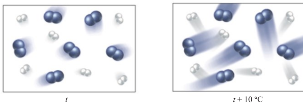
Figura 4.8. Sistemet e reagimit në temperatura të ndryshme.
