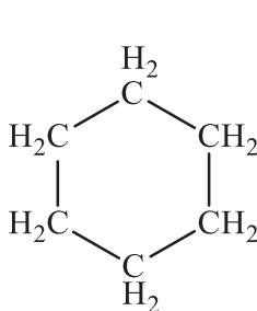
Cikloheksan
