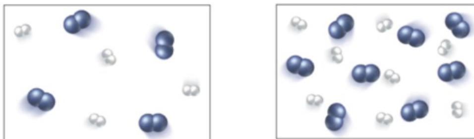
Figura 4.5. Sistemet e reaksionit me përqëndrime të ndryshme të reaktantëve.
