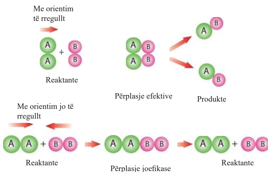
Figura 4.4. Një shembull i përplasjes efektive dhe joefektive.
