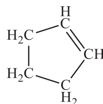
Ciklopentene
