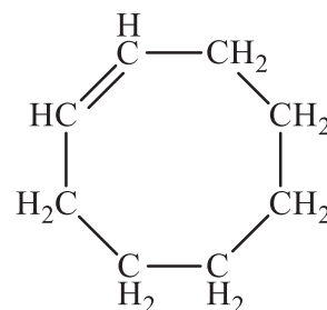
Ciklookten
