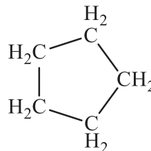
Ciklopentani
