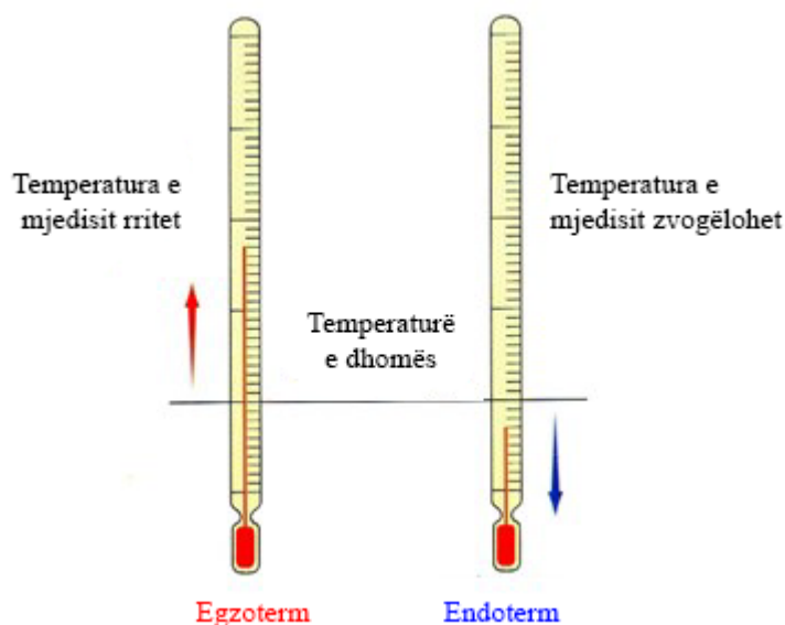
Fig 3.3. Ndryshimet e temperaturës së mjedisit gjatë proceseve egzoterme dhe endoterme.
