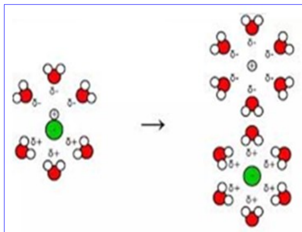
Figura 2.13. Tretja e HCl në ujë dhe hidratimi në ujë dhe të joneve që fitohen.
