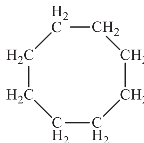
Ciklooktan
