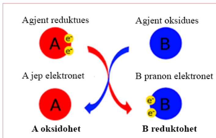
Fig. 6.1 Paraqitja skematike e proceseve redokse
