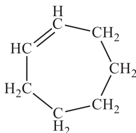
Ciklohepten
