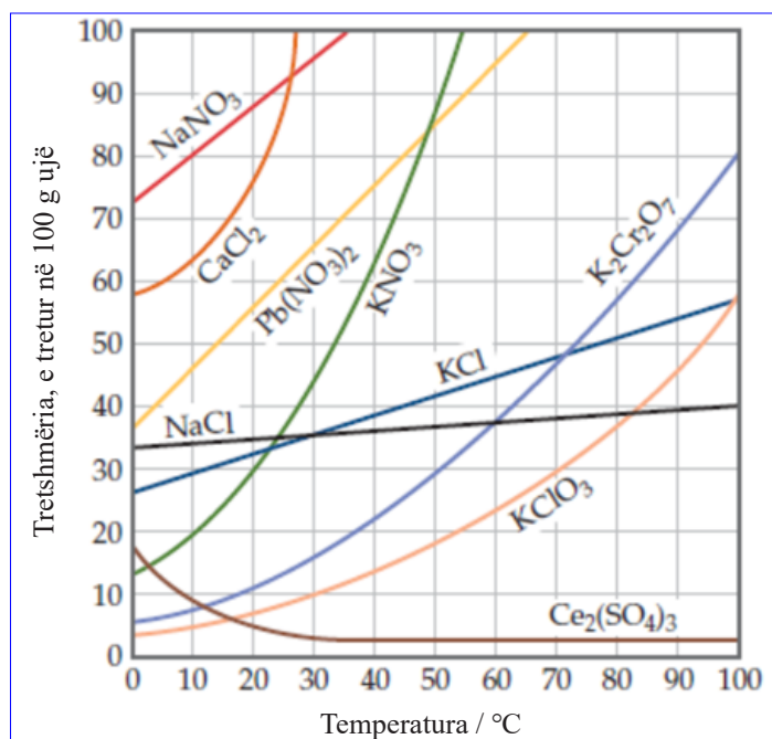
Fig. 2.6. Lakoret e tretshmërisë të substancave të ngurta të ndryshme në ujë
