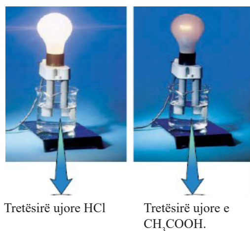
Figura 2.10. Llamba shkëlqen më shumë kur elektodat zhyten në një tretësirë të HCl sesa kur ato zhyten në një tretësirë të \text{CH}_3\text{COOH} .
