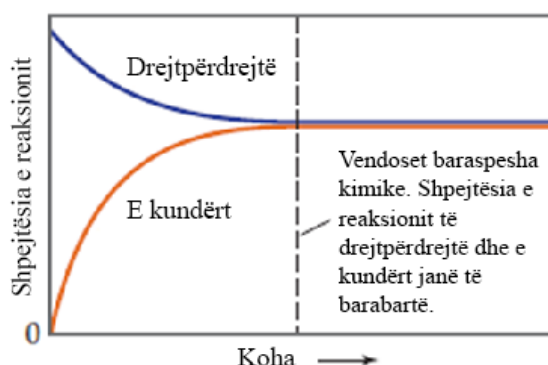
Fig. 5.3. Baraspesha kimike vendoset kur shpejtësia e reaksioneve të drejtpërdrejtë dhe të kundërta bëhen të barabarta.
