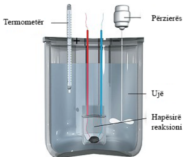
Fig. 3.4. Kolorimetër
